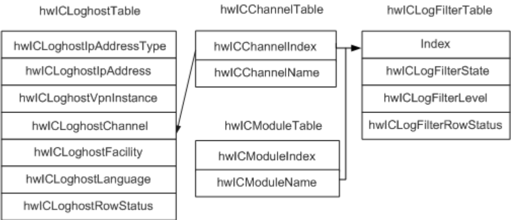
图 59-1 HUAWEI-INFOCENTER-MIB 表间关系图
